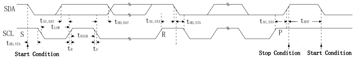
I2C时序图
