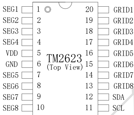
TSSOP20/SOP20
