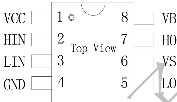
图 2 管脚图
