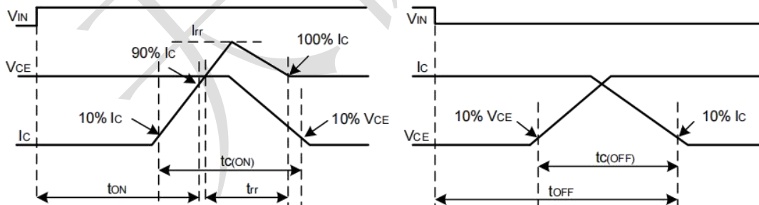
图 3. 开关时间的定义 Figure 3. Definition of switching time
