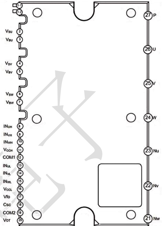
图 2: 引脚定义图
