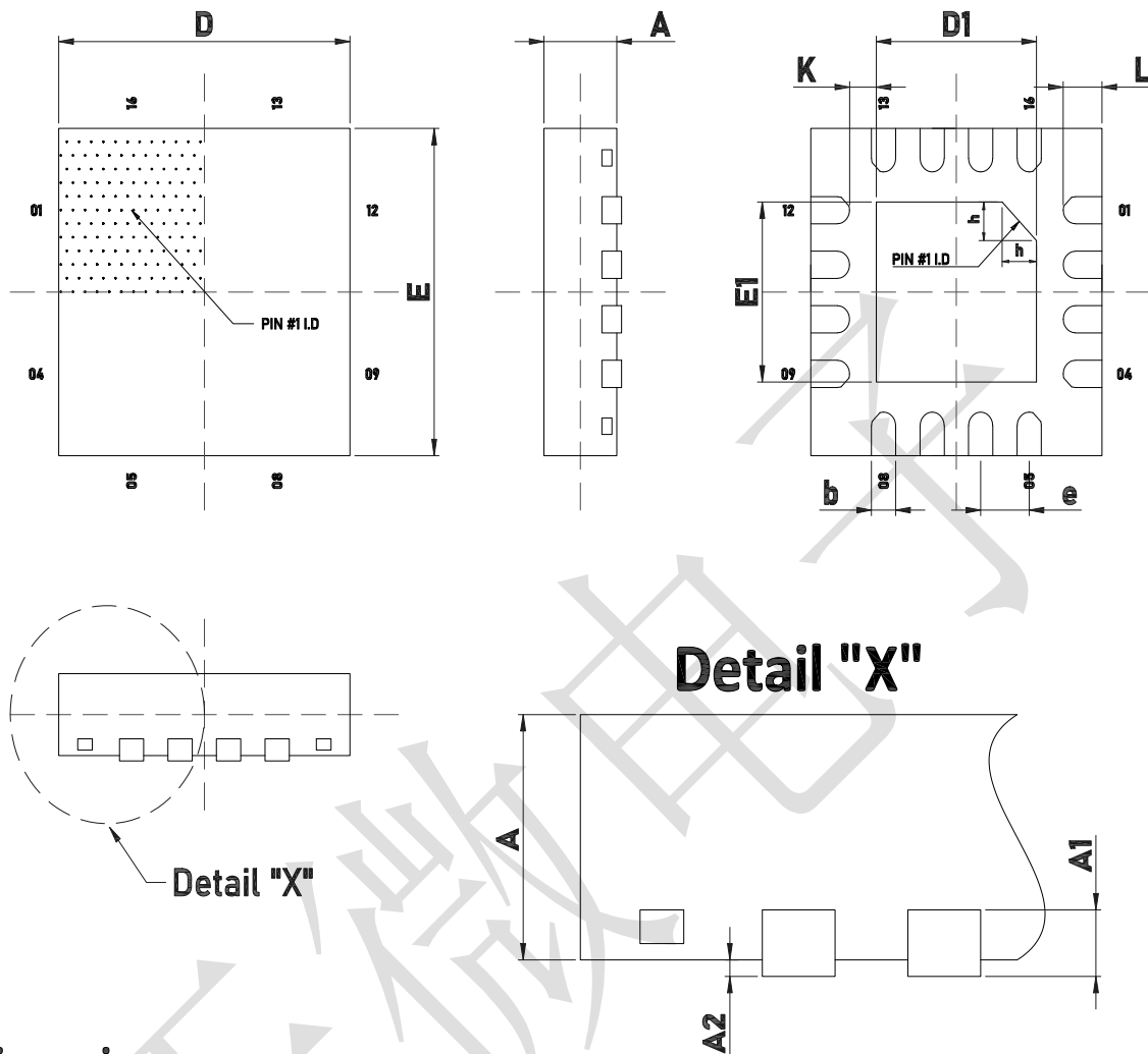
封装示意图 (QFN-16: 3mm × 3mm)
