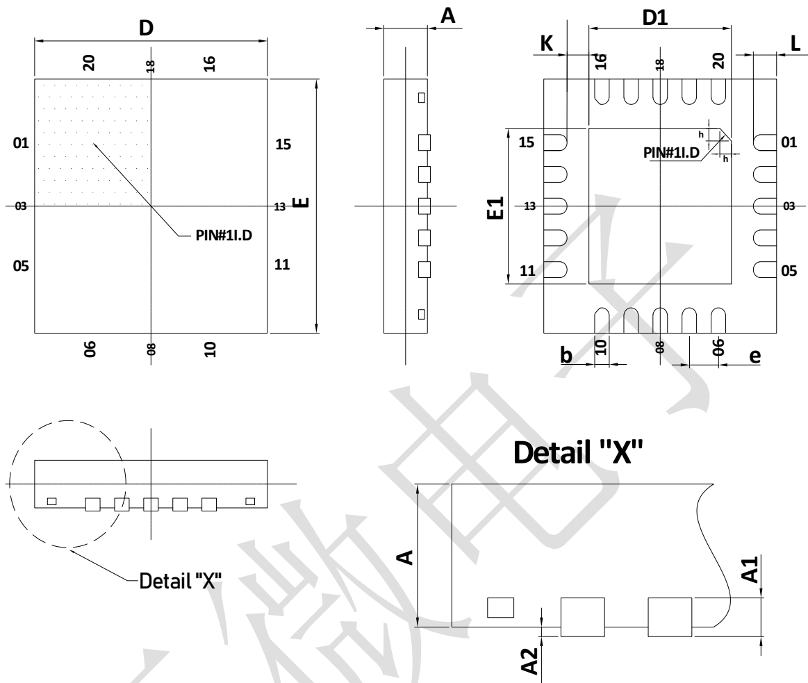
封装示意图(QFN-20:4mm×4mm)
