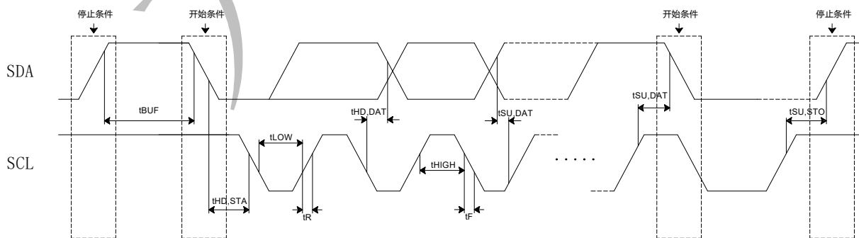
I2C 时序图
