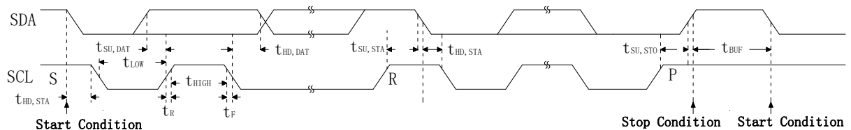
I2C 时序图
