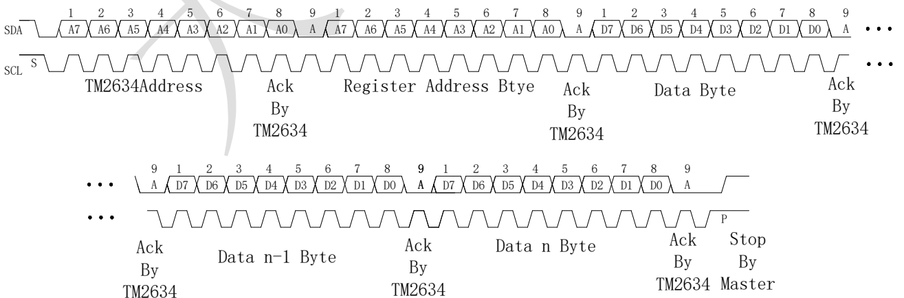
I2C 连续写入时序
