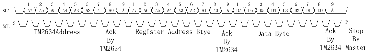
I2C写数据时序
